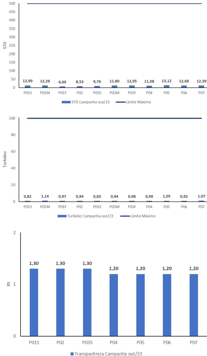
Figura 14. Parâmetros relacionados aos teores de sólidos e compostos dissolvidos nas águas. Nota: (1) Limite da Resolução CONAMA 357/2005 (Classe 2) indicado nos gráficos, quando cabível.
