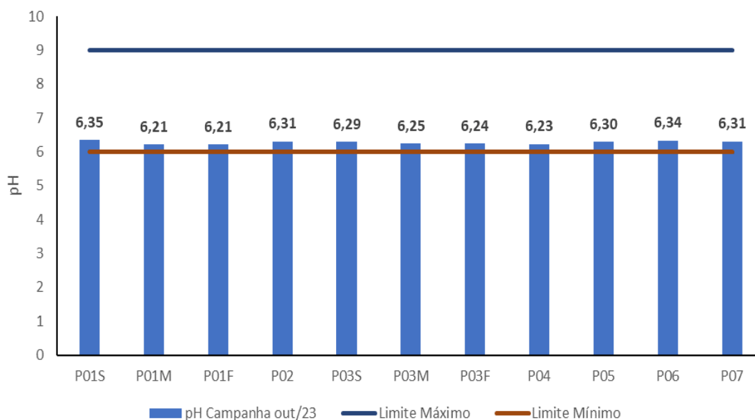
Figura 11. Parâmetros relacionados ao equilíbrio ácido-básico e iônico da água. Nota: (1) Limite da Resolução CONAMA 357/2005 (Classe 2) indicado nos gráficos, quando cabível.
