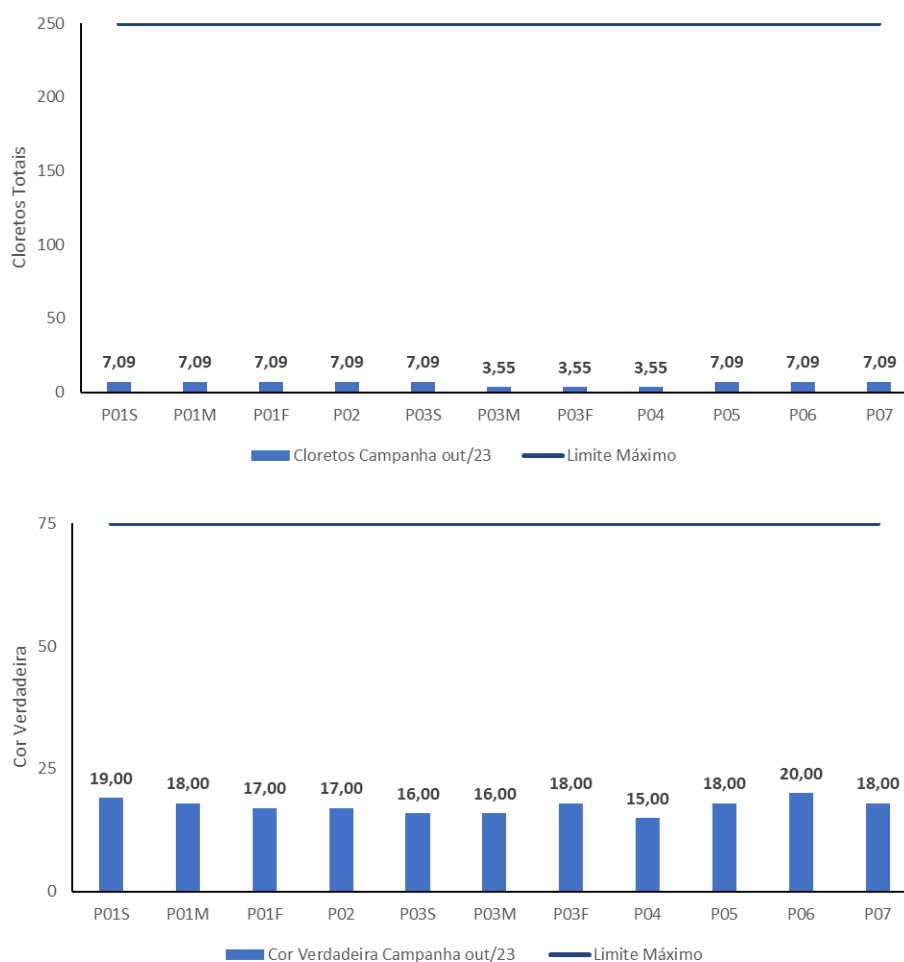
Figura 16. Parâmetros relacionados aos compostos dissolvidos nas águas. Nota: (1) Limite da Resolução CONAMA 357/2005 (Classe 2) indicado nos gráficos, quando cabível.
