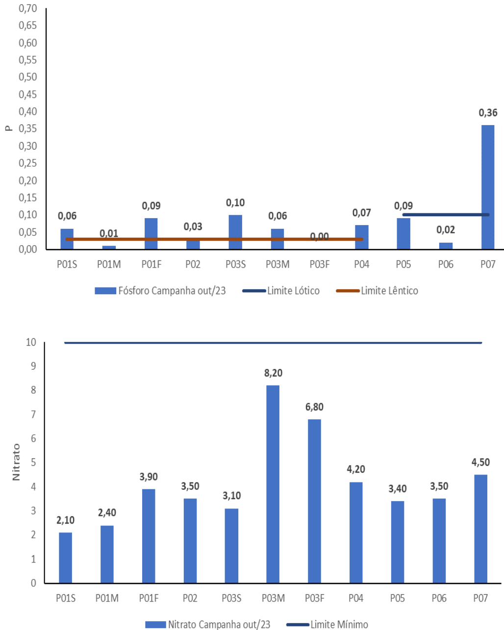
Figura 12. Parâmetros relacionados aos nutrientes dissolvidos na água. Nota: (1) Limite da Resolução CONAMA 357/2005 (Classe 2) indicado nos gráficos, quando cabível.
